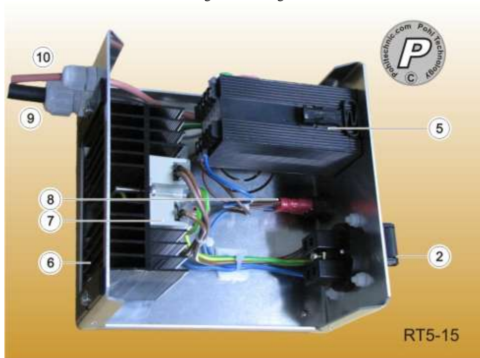
Verdrahtungsansicht Regler RT5-15
